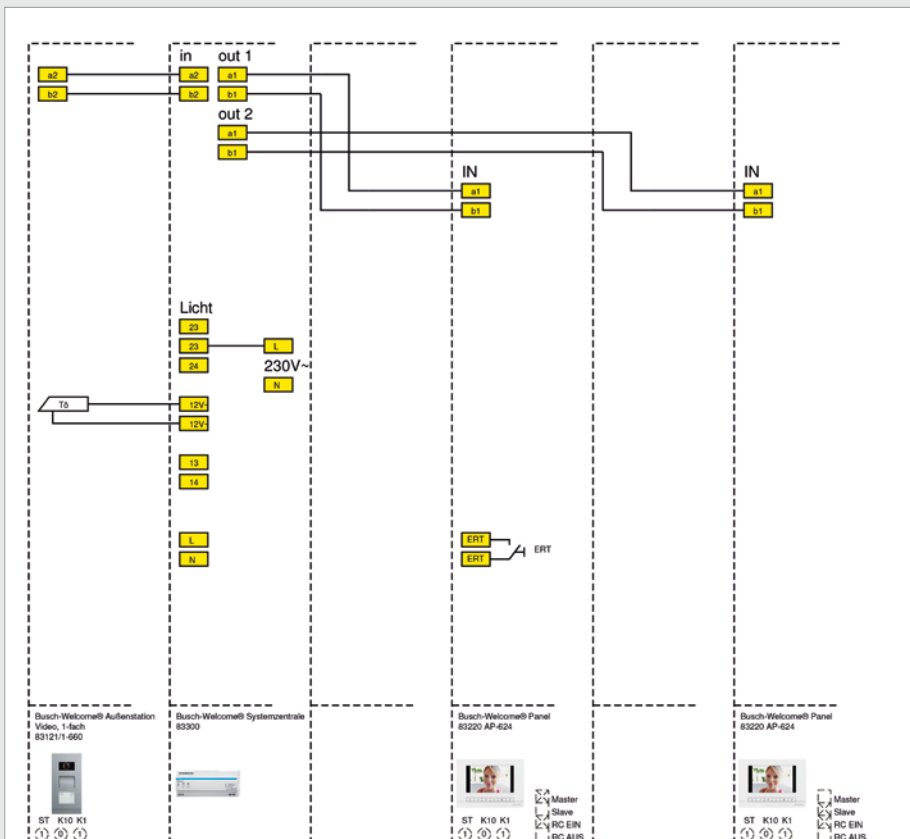
Außenschaltplan
