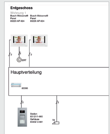
Übersichtsverbindungsplan
